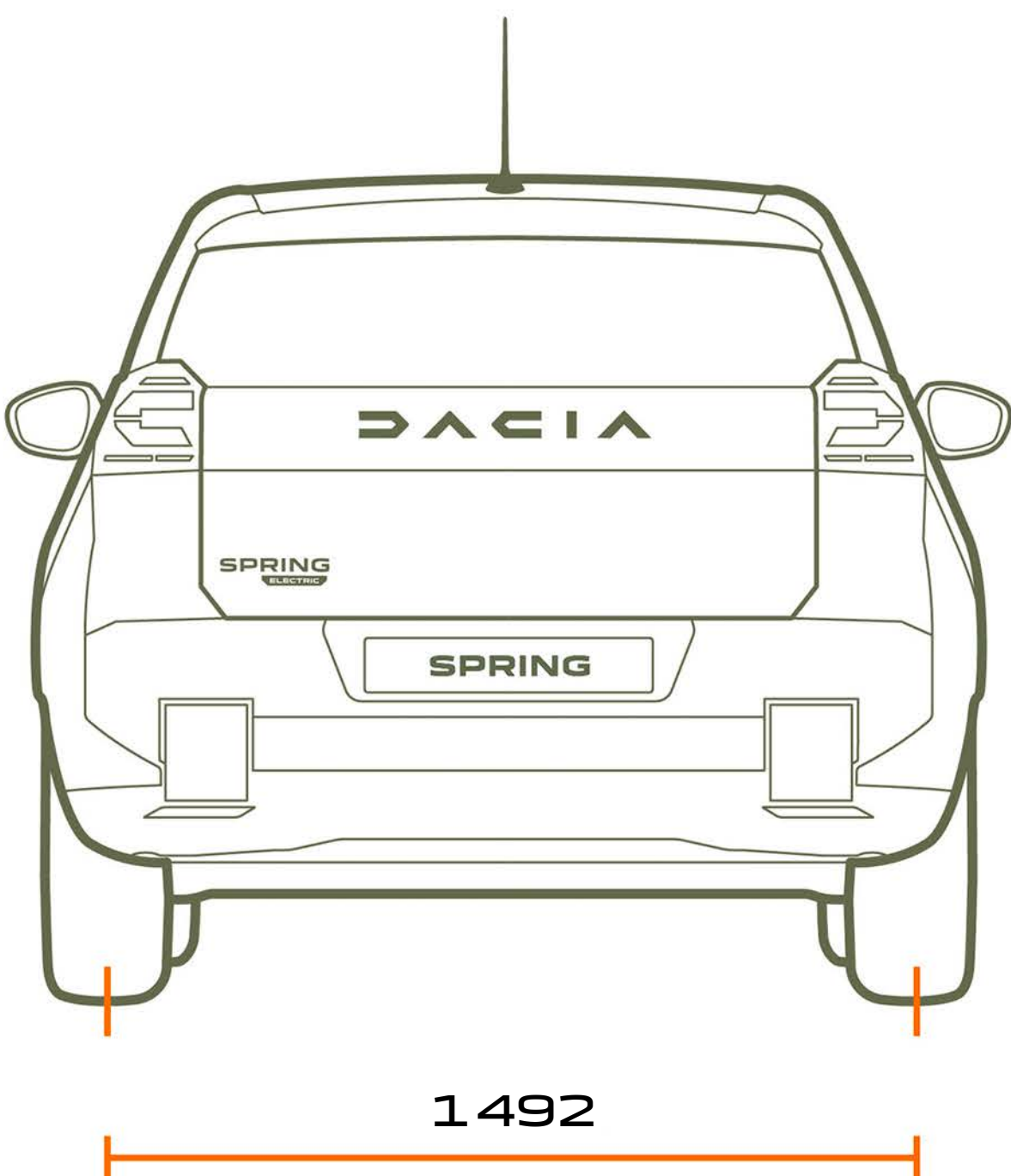
VUE ARRIÈRE
