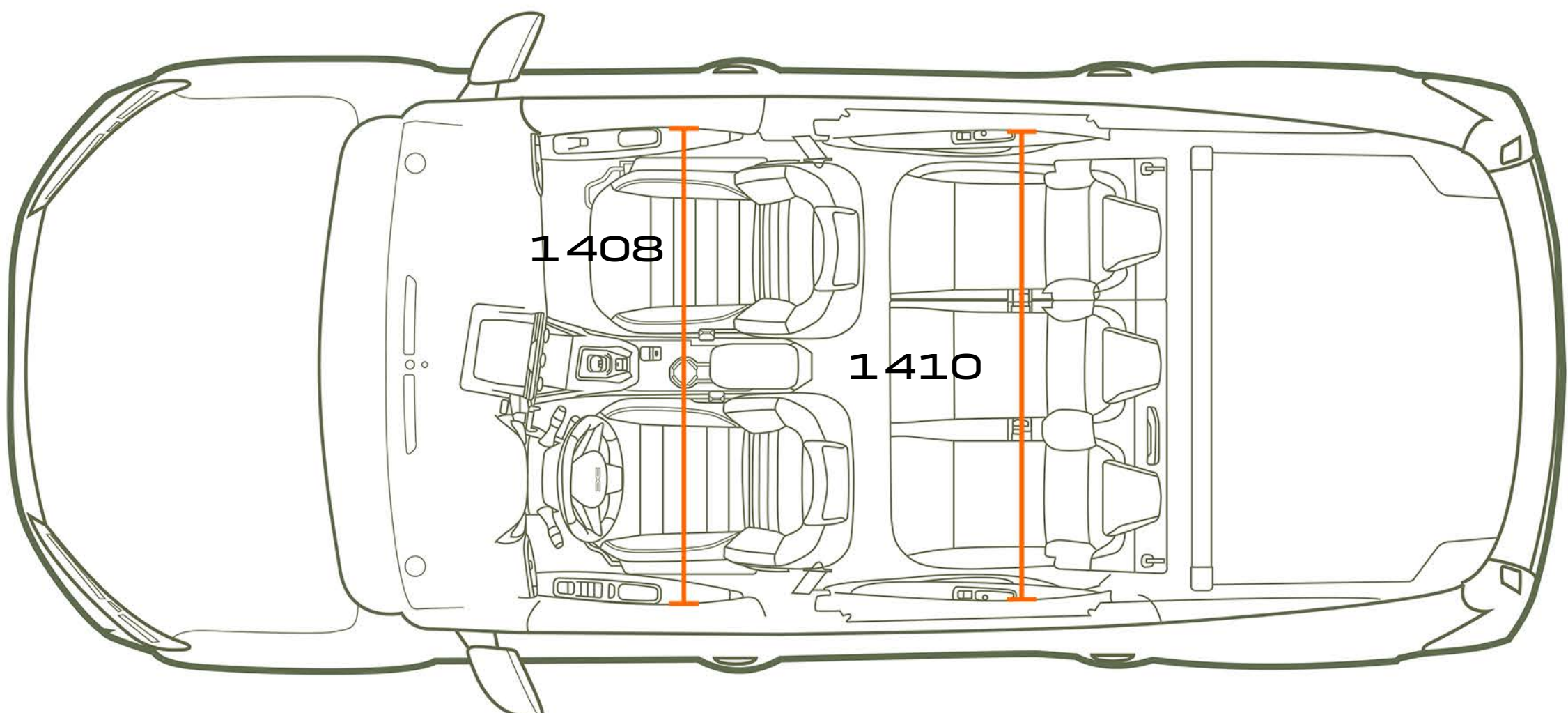
VUE DE DESSUS 5 PLACES
