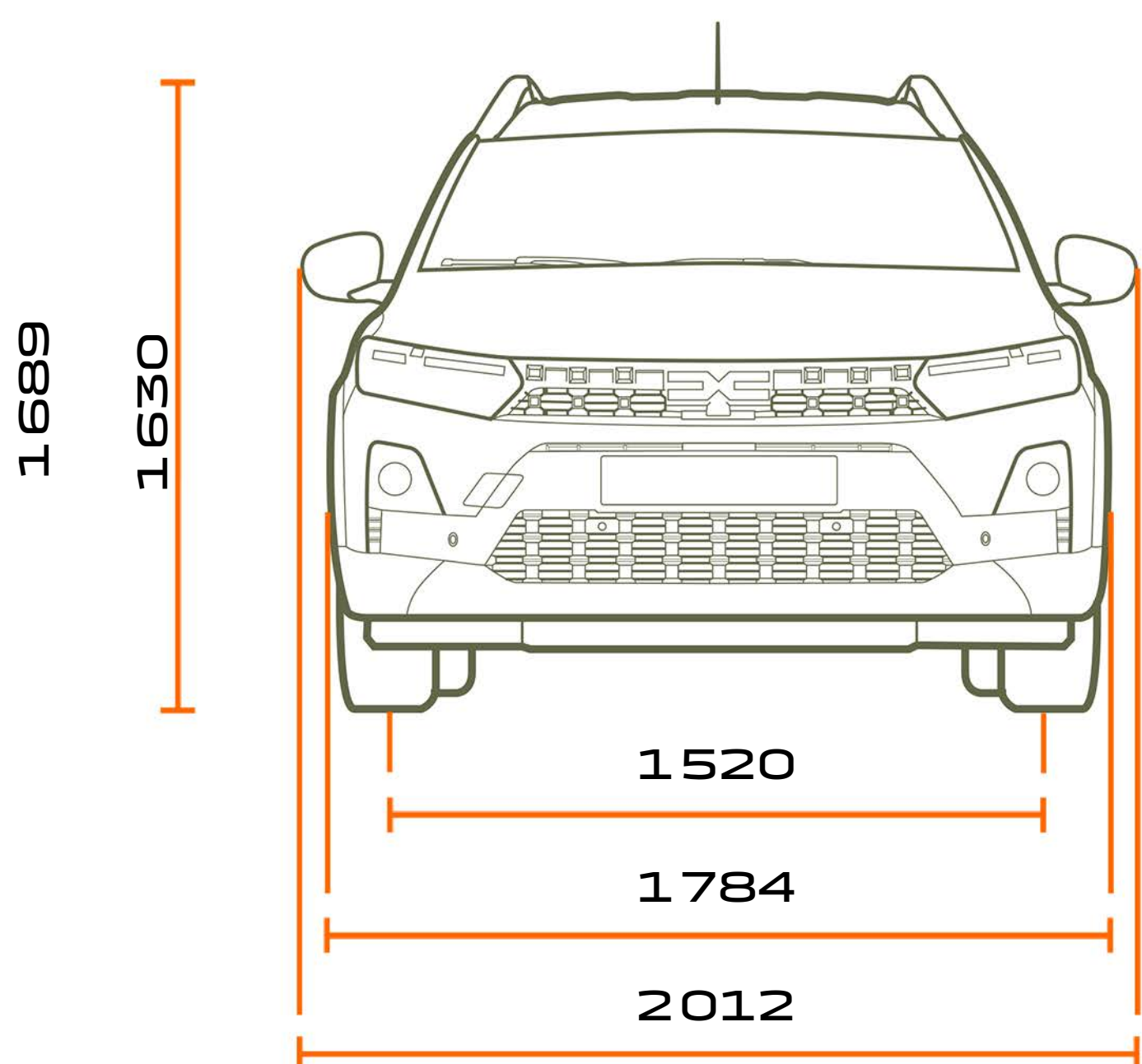
VUE AVANT 5 ET 7 PLACES
