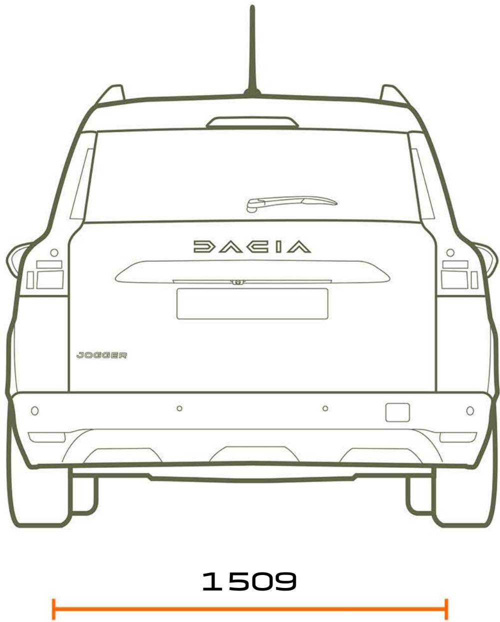
VUE ARRIÈRE 5 ET 7 PLACES
