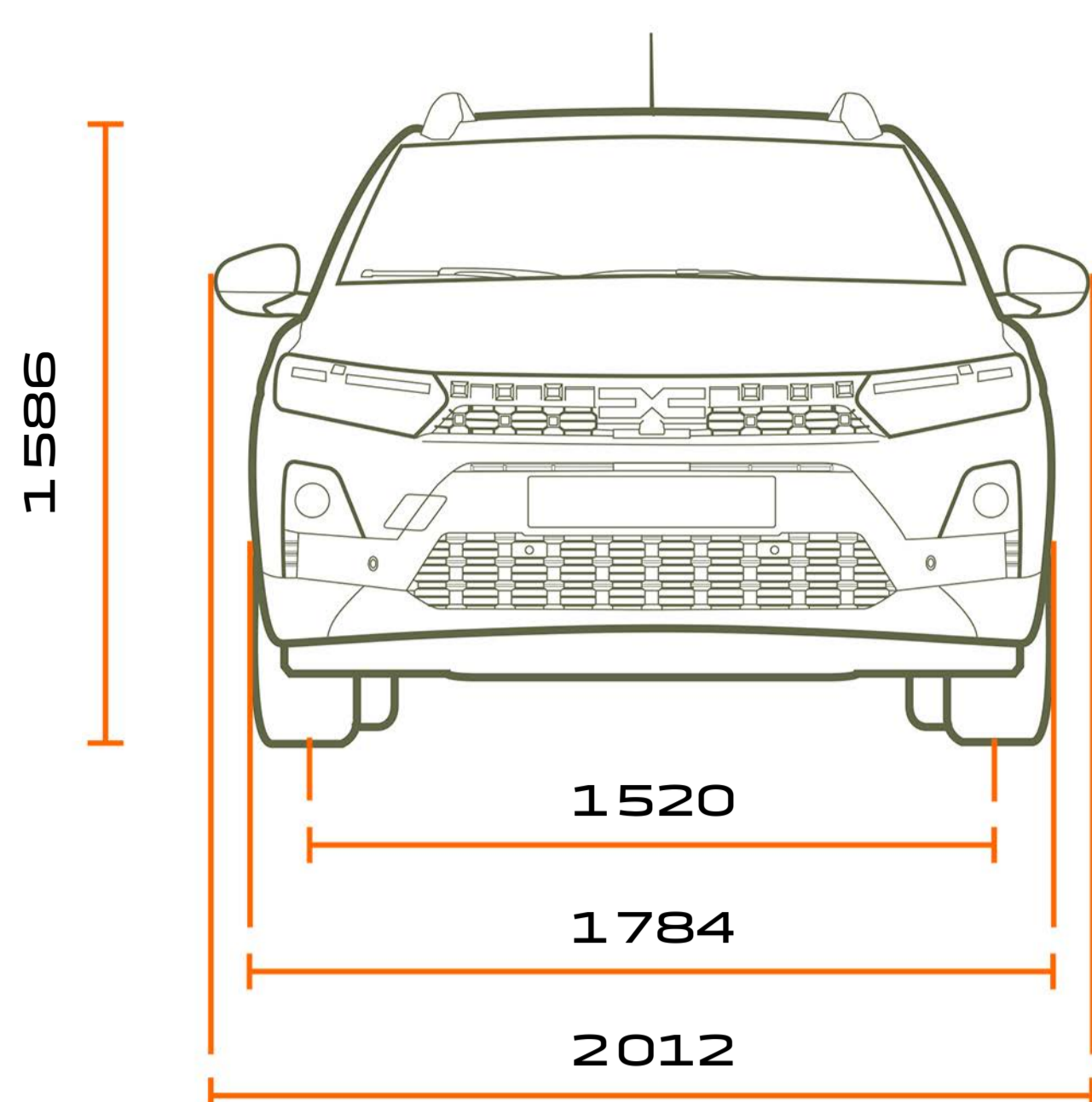
VUE AVANT
