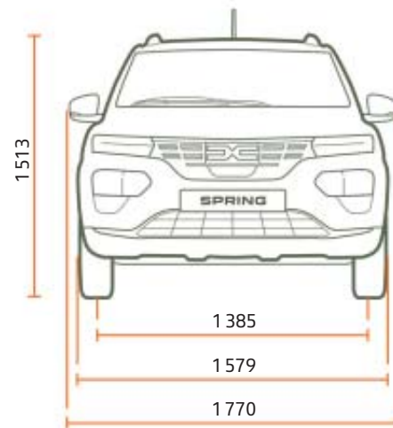
VUE AVANT
